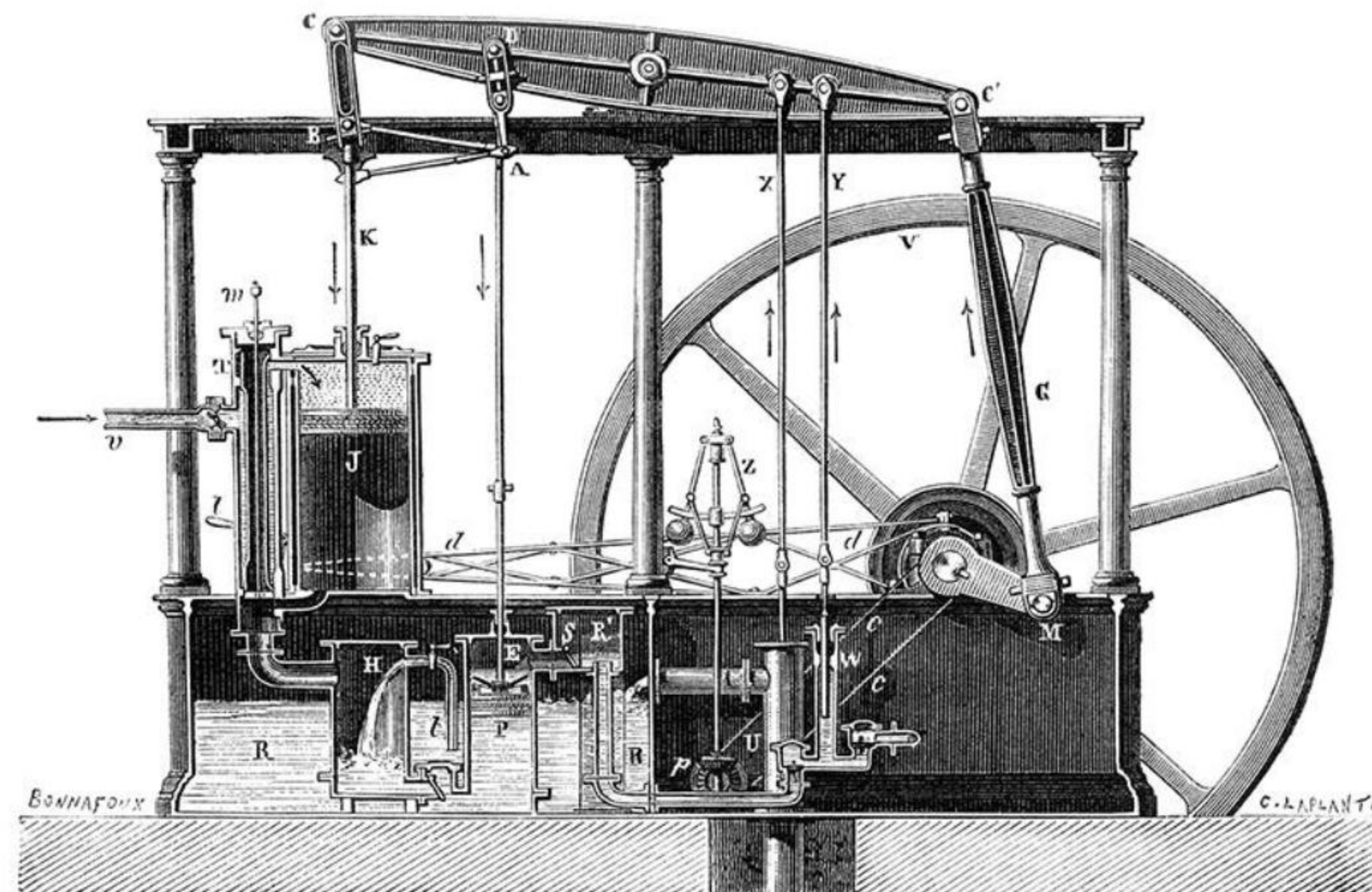
Fig. 59. — Machine à balancier de Watt.
